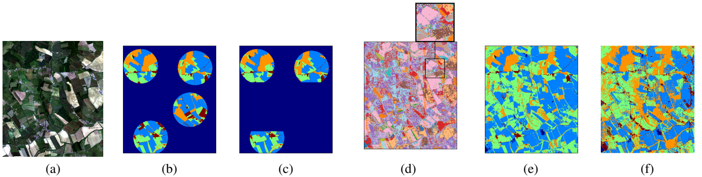
FIGURE 2 – (a) Composition colorée de l’image réelle, (b) vérité terrain, (c) vérité terrain pour l’entraînement, (d) clusters estimés, (e) classification réalisée par le modèle proposé, (f) classification réalisée avec un modèle gaussien.
